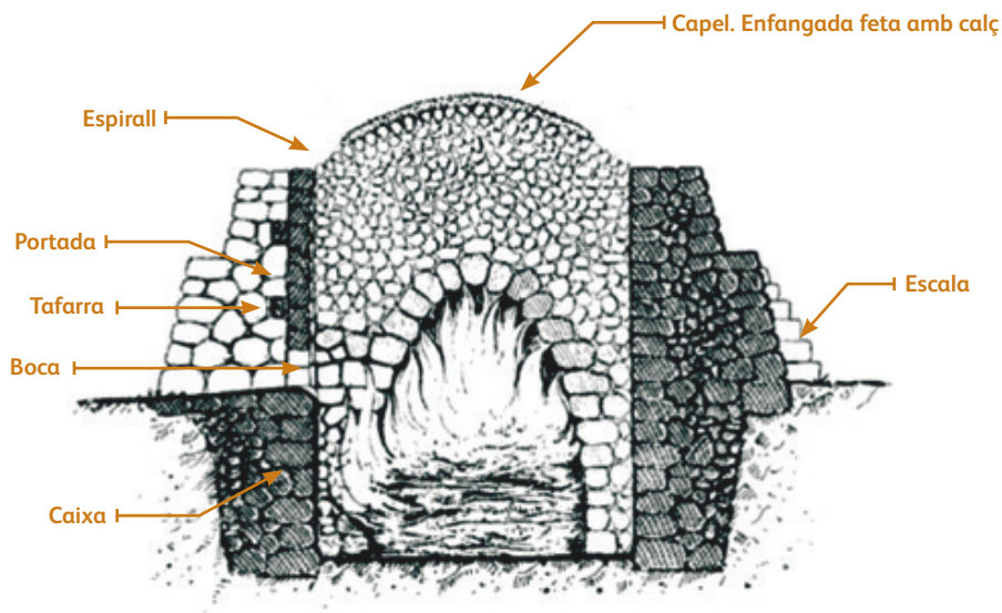
Forn de calç, segons dibuix de Miquel Fullana al Diccionari de l'Art i dels Oficis de la Construcció.
